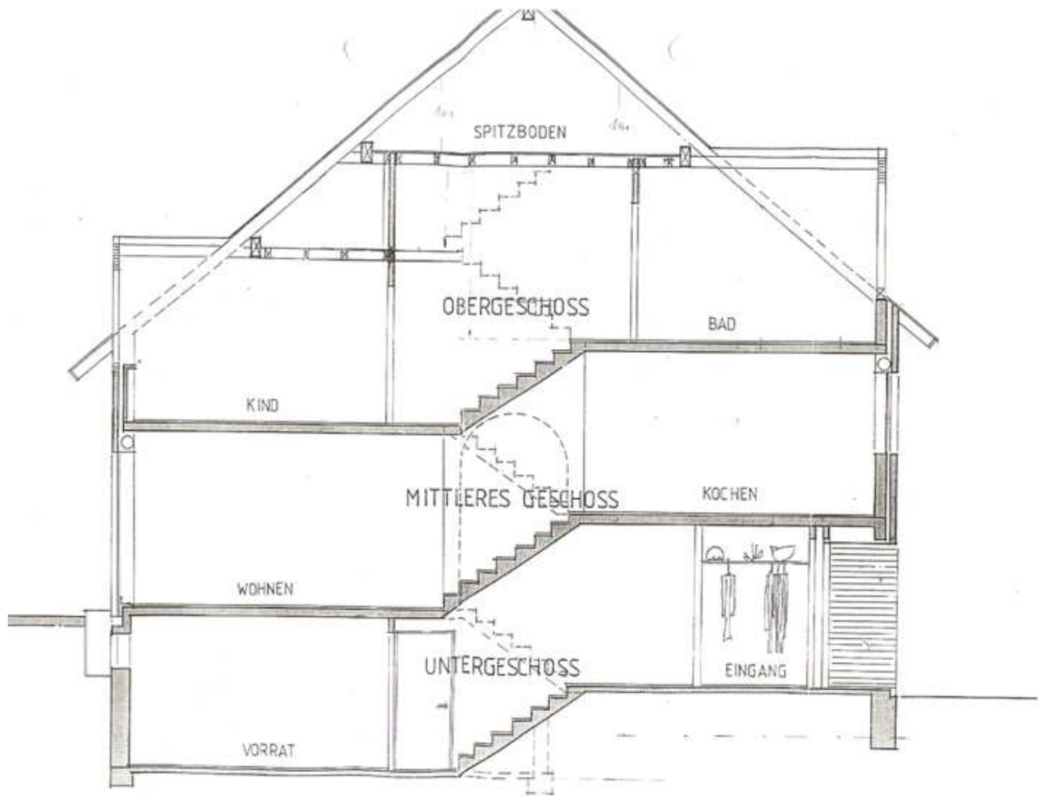
SCHNITT M 1:50
